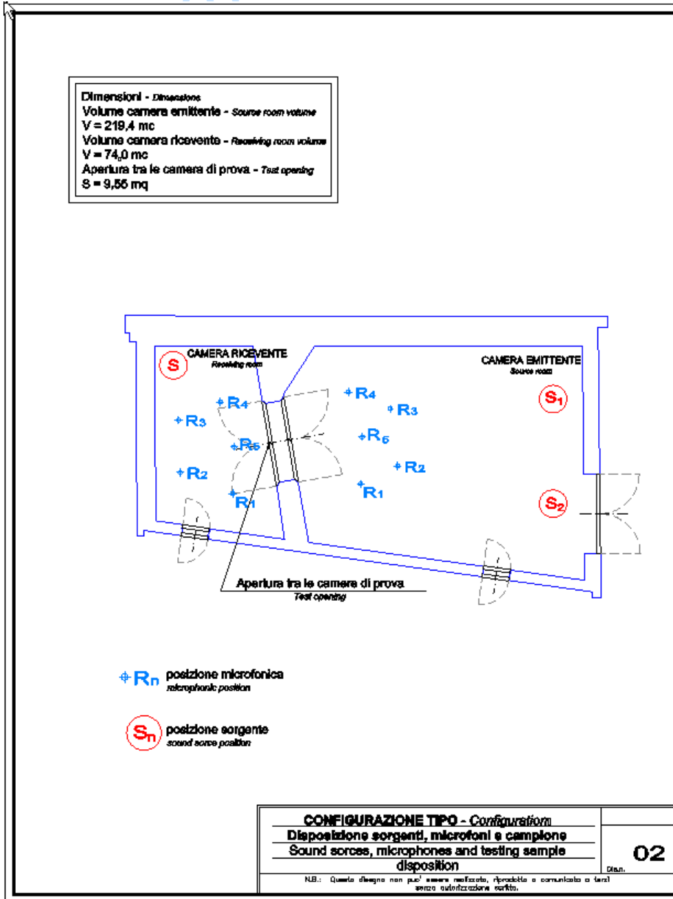
Figura 2: Planimetria della camera di prova Figure 2: Drawing of the test rooms
